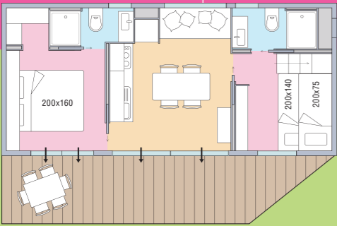
VERZASCA LODGE 5 34,4 m 2 + 21 m 2 Terrasse max. 5 Personen, min. 2 Person
