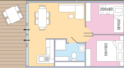
IGLOO TUBE 37.7 m 2 + 12.5 m 2 Terrasse max. 4 Personen, min. 2 Person Nr. 433 – 437
